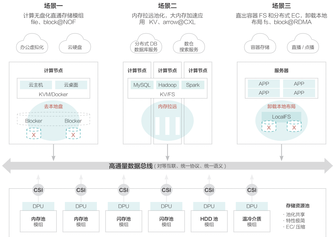
图 3-9 存算分离架构
