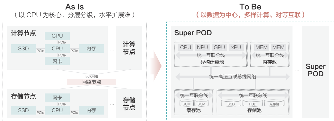
图 4-3 以数据为中心的多样算力系统参考架构
